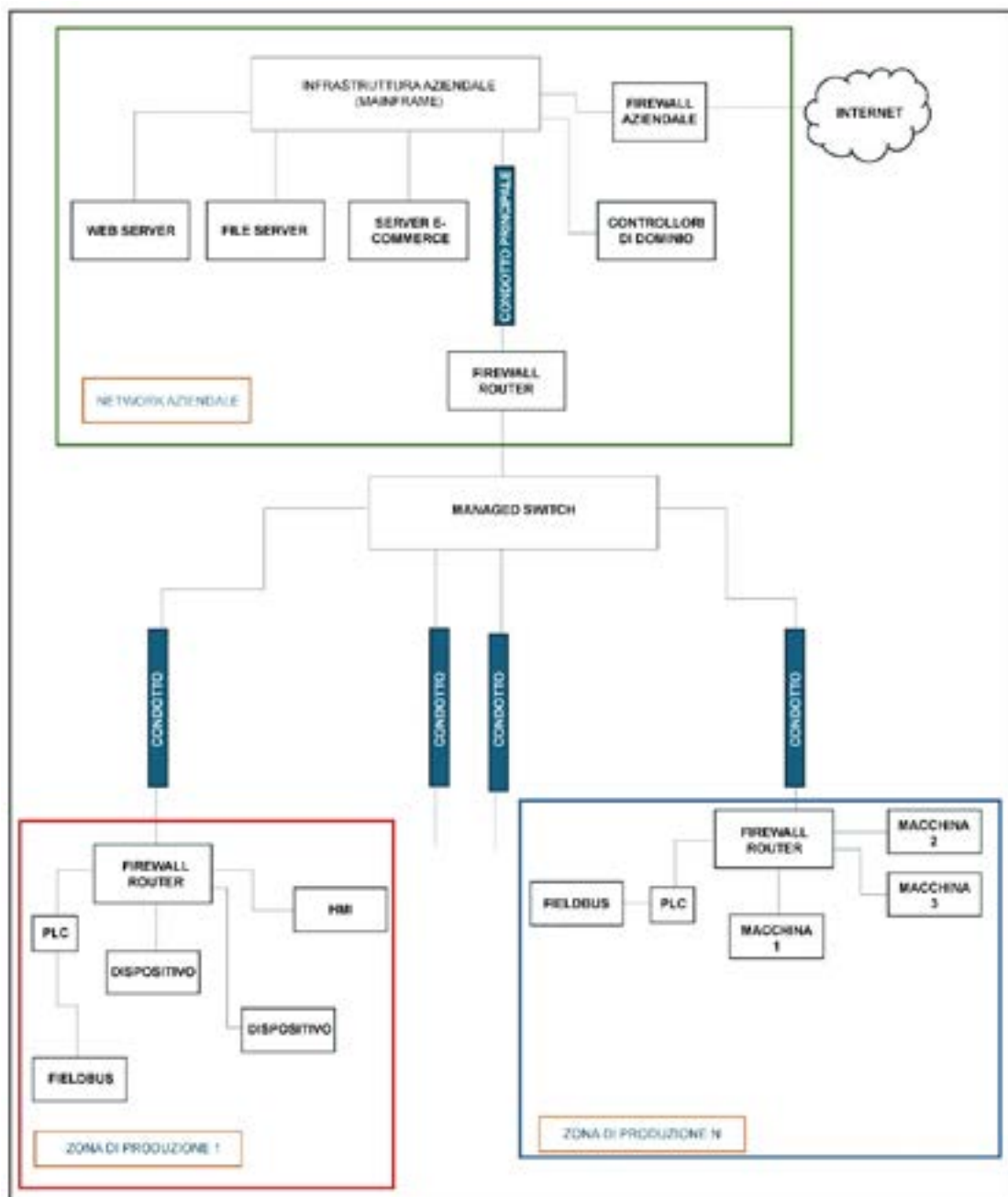
Figura 2: Rappresentazione dei principali processi industriali manifatturieri
